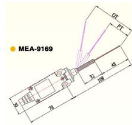
MEA-9169 Plastic mini limit switch, MEA-9169G Plastic mini limit switch, flat tail
