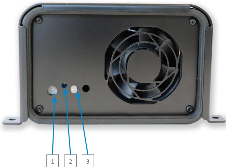
Abb. 1: ABC Frontansicht
